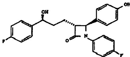
Ezetimibe
